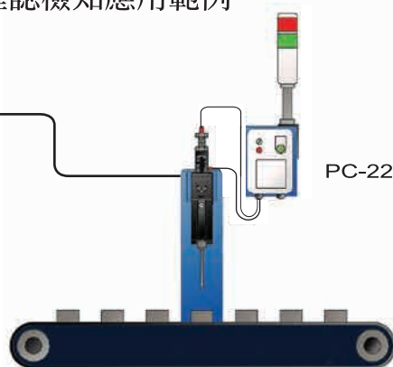
吐油確認檢知及備油確認檢知應用範例
