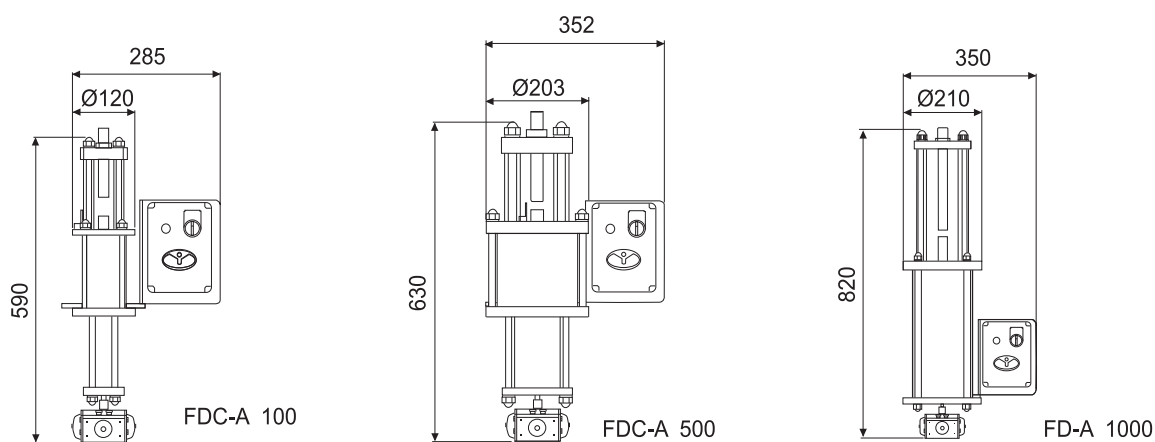
定量缸配置圖
